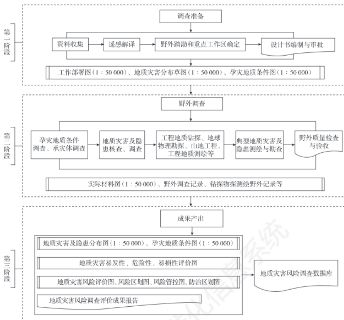
图 1 地质灾害风险调查评价流程图
