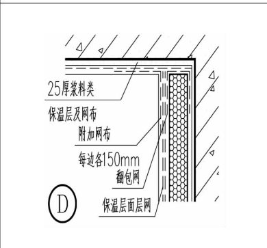
K.0.10 开敞式阳台节点
