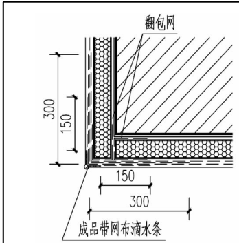
K.0.13 滴水线部位构造
