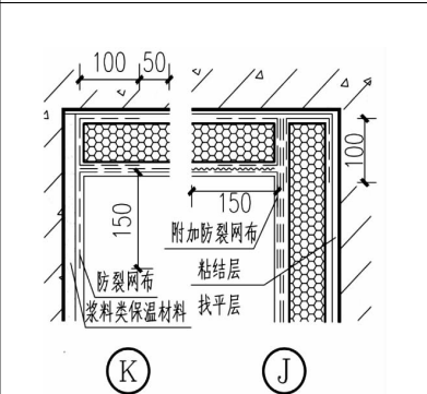
K.0.28 节点构造
