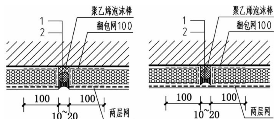
a. 明缝做法 b. 暗缝做法 1、聚乙烯泡沫棒 2、硅酮建筑密封胶
