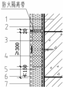
1—基层墙体；2—界面剂；3—聚合物水泥防水砂浆找平防水层、胶粘剂； 4—防火隔离带保温板；5—保温板； 6—耐碱玻纤网布+附加抗裂耐碱玻纤网布；7—饰面材料
