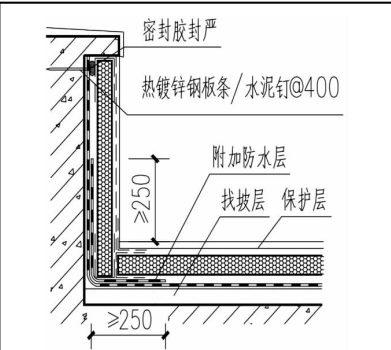
K.0.26 倒正式非上人屋面与女儿墙节点
