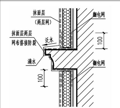
K.0.16 外挑装饰构造(二)
