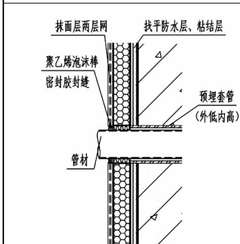
K.0.17 穿墙预埋套管构造
