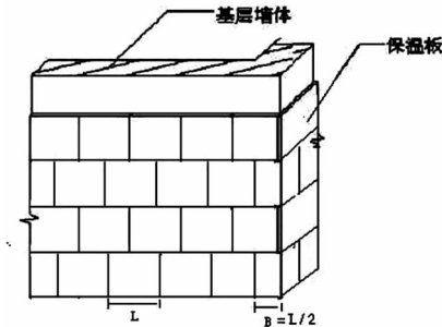
图 6.3.6-1 保温板墙体排板及转角排板示意
