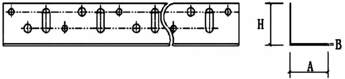
图 4.4.10 铝合金托架示意
