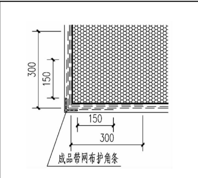
K.0.14 阳角护角条部位构造
