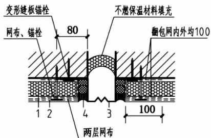
1—保温层;2—保护层(抹面层和饰面层); 3—盖板;4—聚乙烯泡沫棒、密封胶嵌填 图 5.2.4-3 结构变形缝构造示意图
