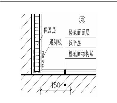
K.0.30 外墙内外组合保温楼地面节点构造
