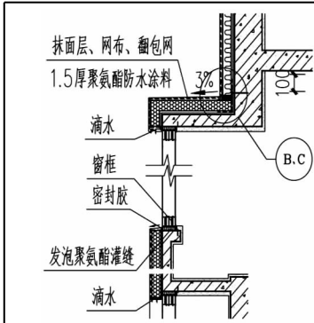
K.0.7 封闭式阳台剖面
