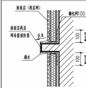
K.0.15 外挑线条构造(一)
