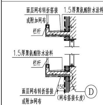
K.0.9 开敞式阳台剖面
