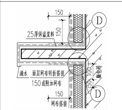
K.0.18 空调外机挑挑板、雨篷
