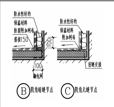
K.0.8 封闭式阳台节点构造
